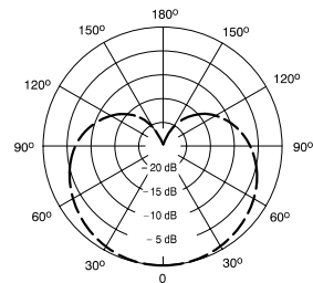
標準指向特性
