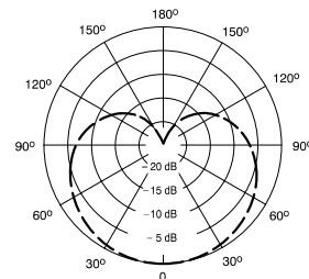
1000 Hz Corak Kutub Khas
