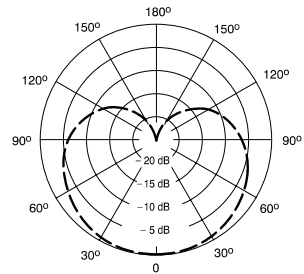
Diagramma polare tipico
