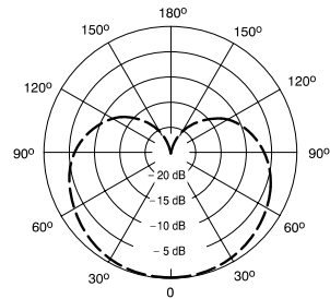
Corak Kutub Khas
