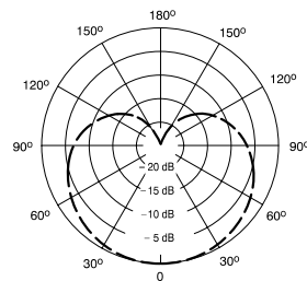
1000 Hz Courbe de directivité typique
