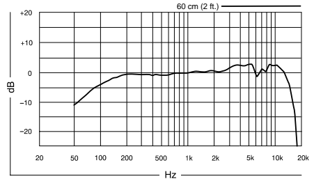
주파수 응답
